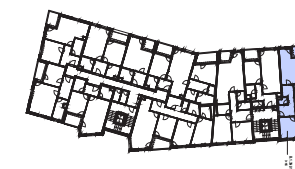
PŮDORYS PATRA
