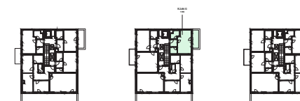
PŮDORYS PATRA
