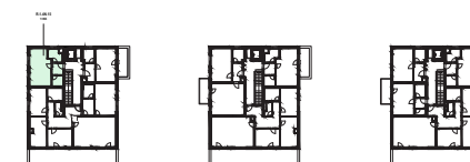
PŮDORYS PATRA
