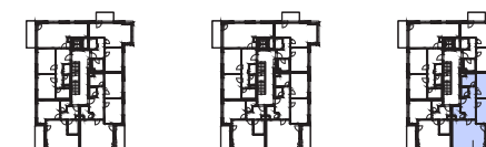
PŮDORYS PATRA
